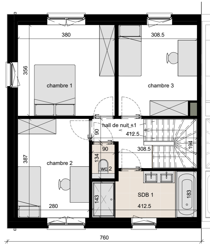
étage surf. brute 63.46 m 2
