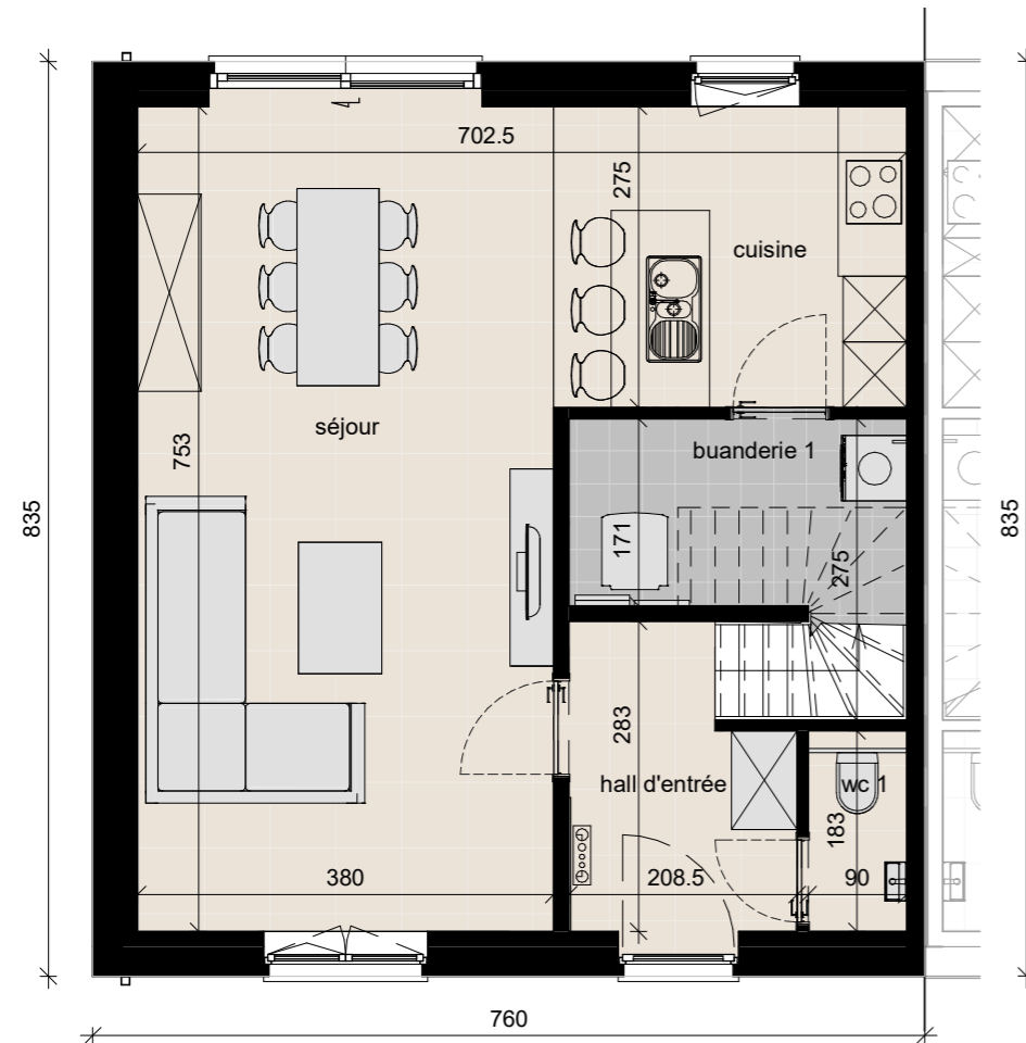
rez-de-chaussée surf. brute 63.46 m 2
